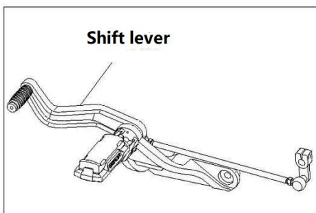
Fig14 Shift position
